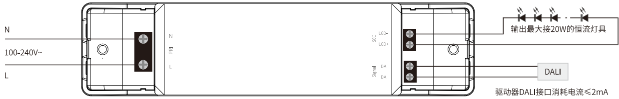
DALI应用接线图
