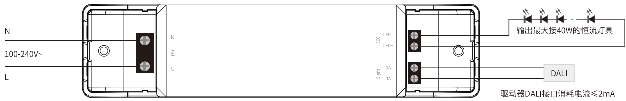
DALI应用接线图
