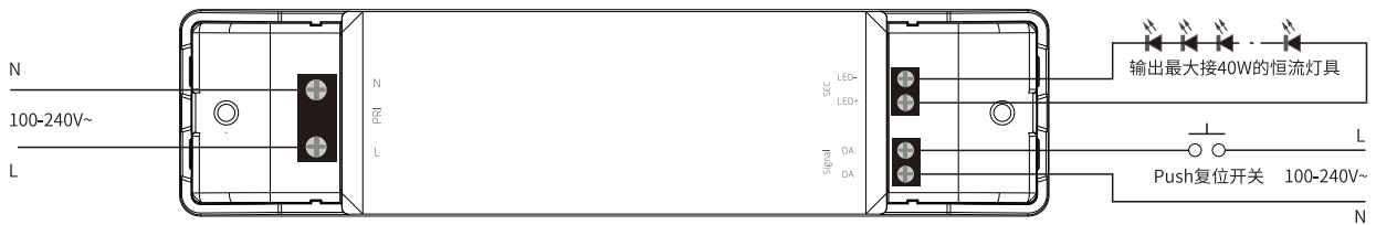
Push DIM应用接线图
