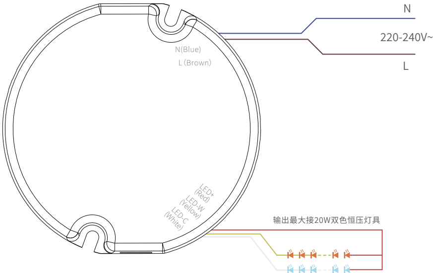
接线图
