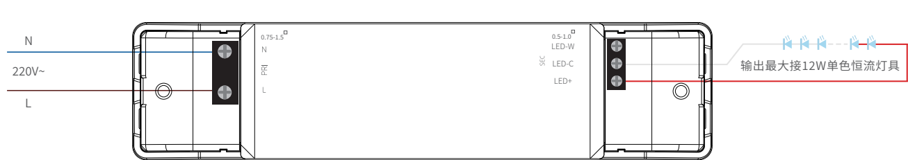
单色模式应用接线图
