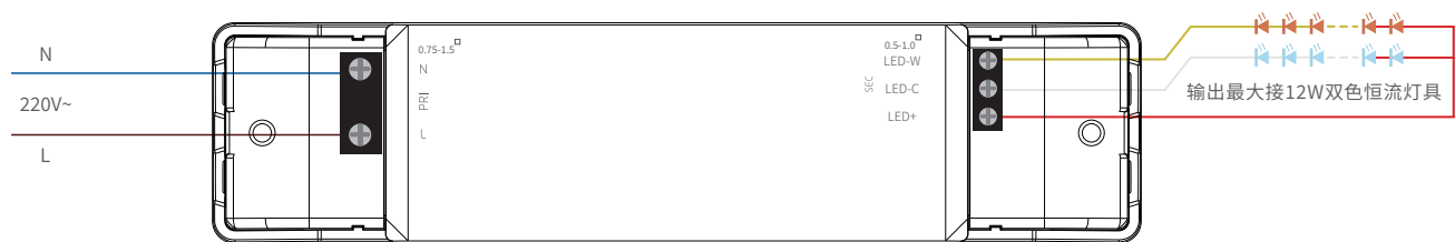
双色模式应用接线图
