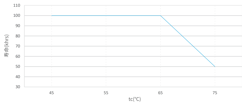
寿命VS温度关系图
