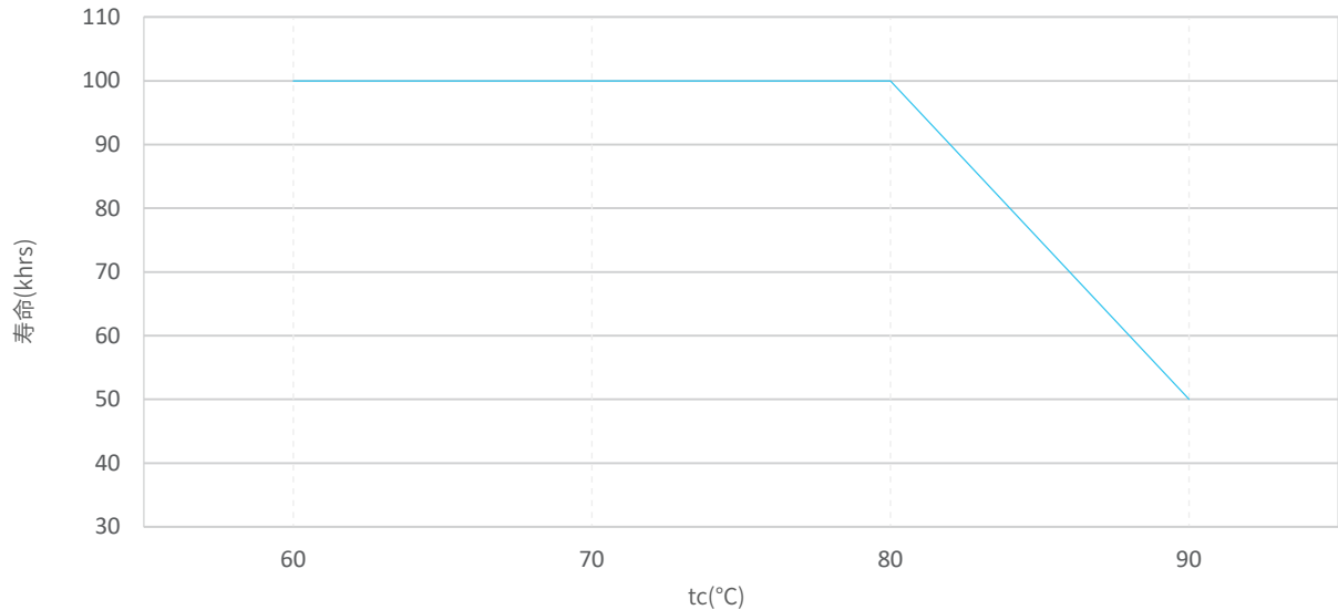
寿命VS温度关系图
