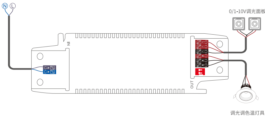
接线图
